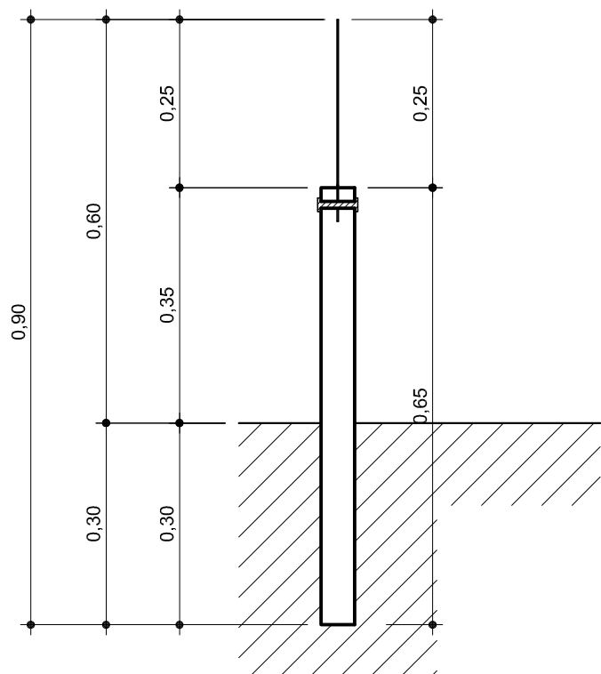
CORTE esc.: 1:10
