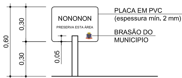
VISTA FRONTAL esc.: 1:20
